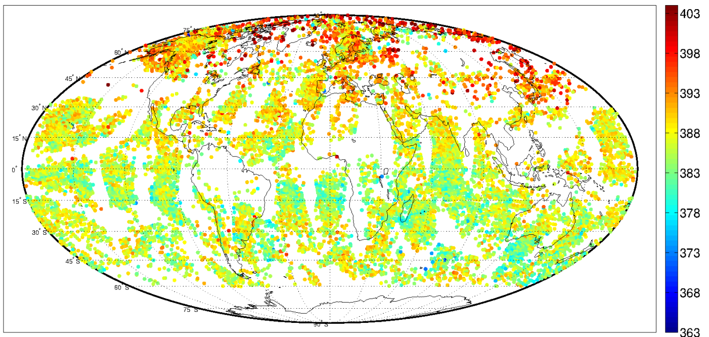
Messdaten zur atmosphärischen CO 2 -Konzentration für Januar 2009
